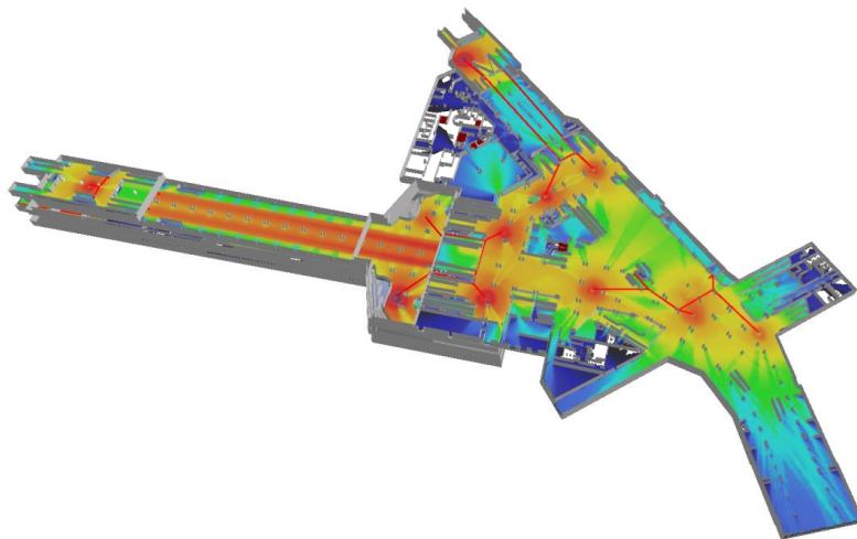
Abbildung 12: Inhouse-Versorgungssimulation (Beispiel)
