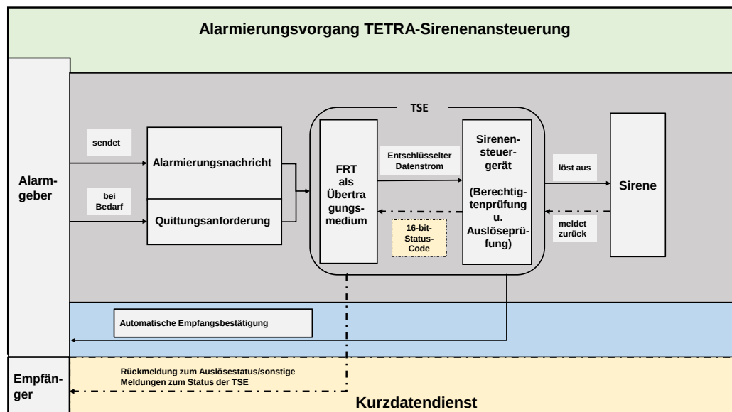
Abbildung 2: Alarmierungsvorgang für die Sirenenansteuerung.
