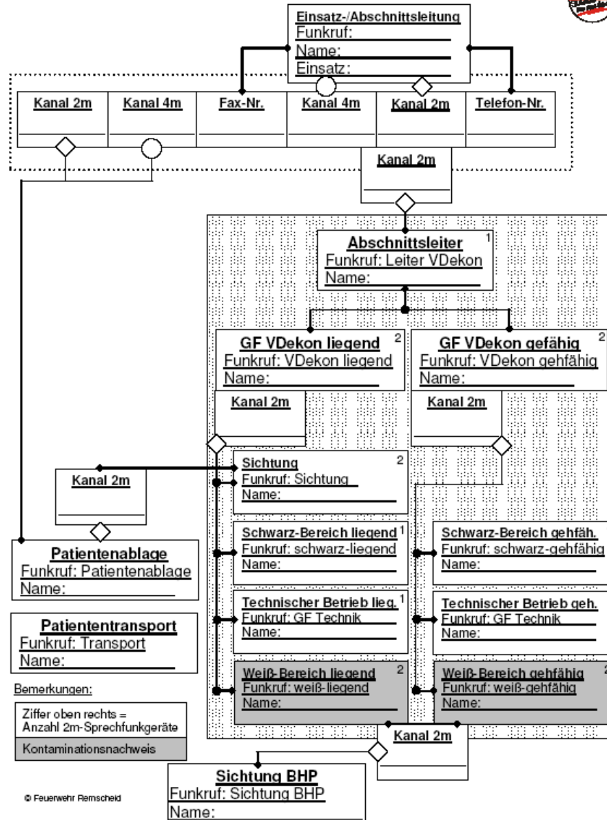
Funkskizze V-Dekon „Überörtlicher Einsatz“
